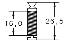
Vorderansicht / Rückansicht / Seitenansicht front view / back view / side view
