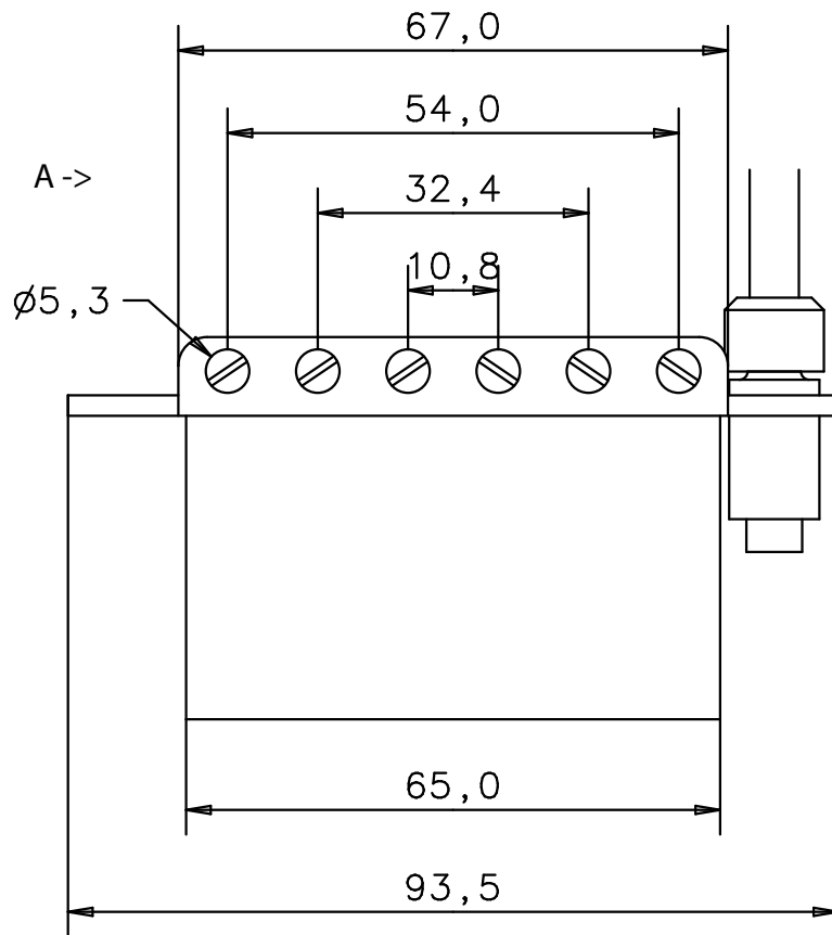
Vorderansicht front view
