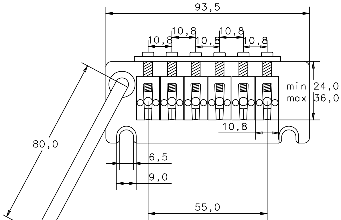
Draufsicht top view
