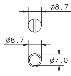
Draufsicht / Untersicht top view / bottom view
